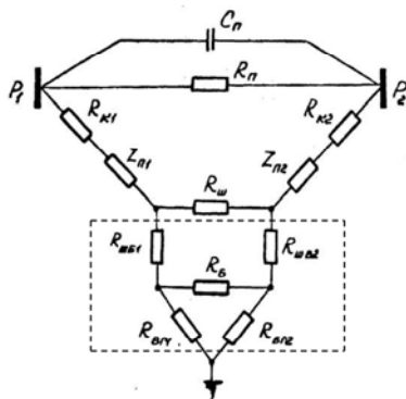
Рис. Схема заміщення опору ізоляції рейкової лінії
