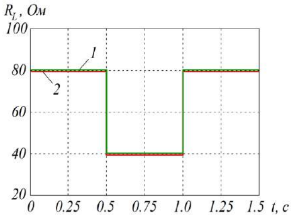
Рис. 10. Спостерігач опору навантаження:
