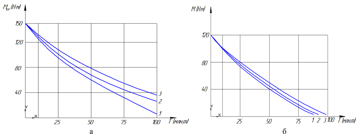
Рис. 1. Графики зависимостей натяжения гаек (а – клеммных, б – закладных) болтов от количества перевезенного груза: 1 – осевые нагрузки более 343 кН; 2 – осевые нагрузки 265-343 кН; 3 – осевые нагрузки до 265 кН
