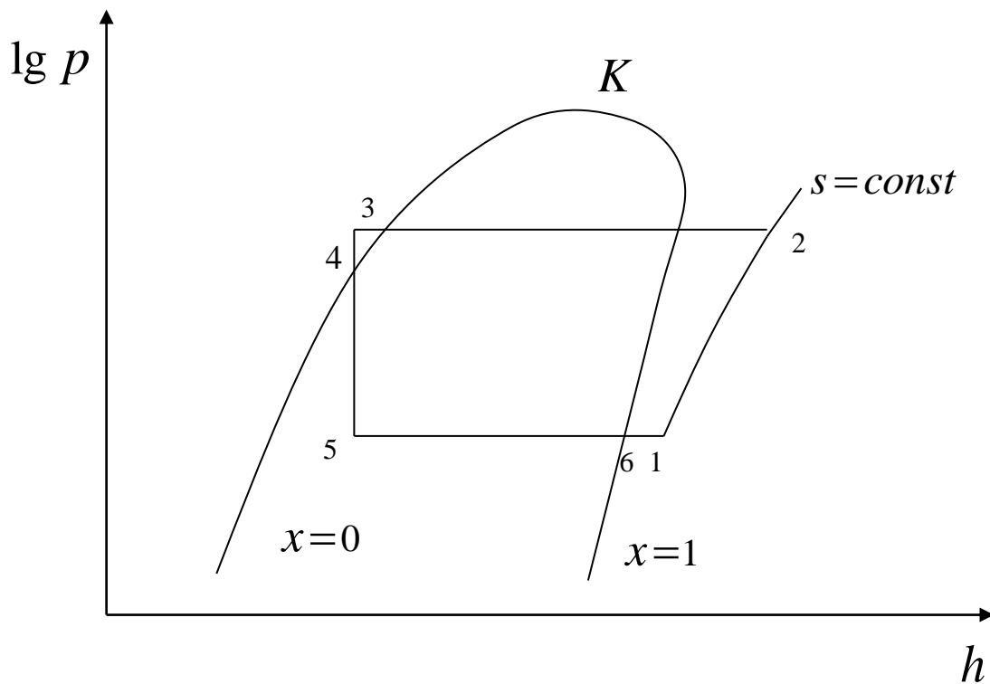
Рисунок 3.1 – Цикл холодильної установки
