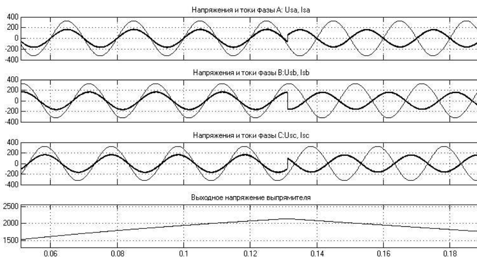
Рис.3 – Осциллограммы фазных токов и напряжений при переходе из режима активного выпрямления в режим рекуперации
