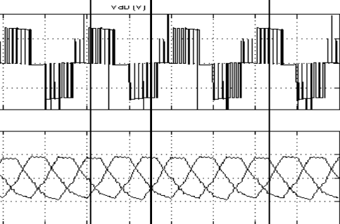
Рис. 8. «Гнучка» структура: пуск, послідовне з'єднання фаз, 1-й рівень регулювання напруги із ШІМ
