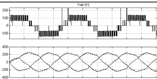
Рис. 10. «Гнучка» структура на 2-му рівні із ШІМ
