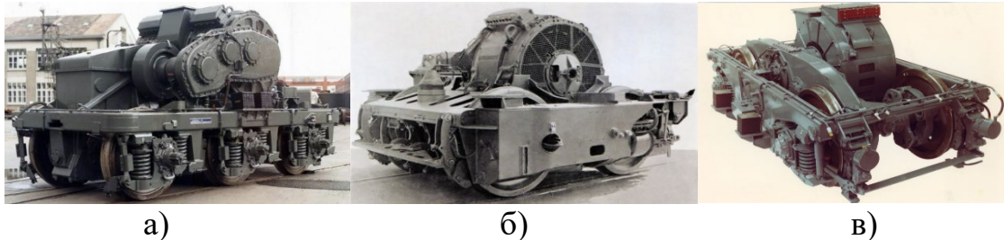
Рис.1. Мономоторні візки:
