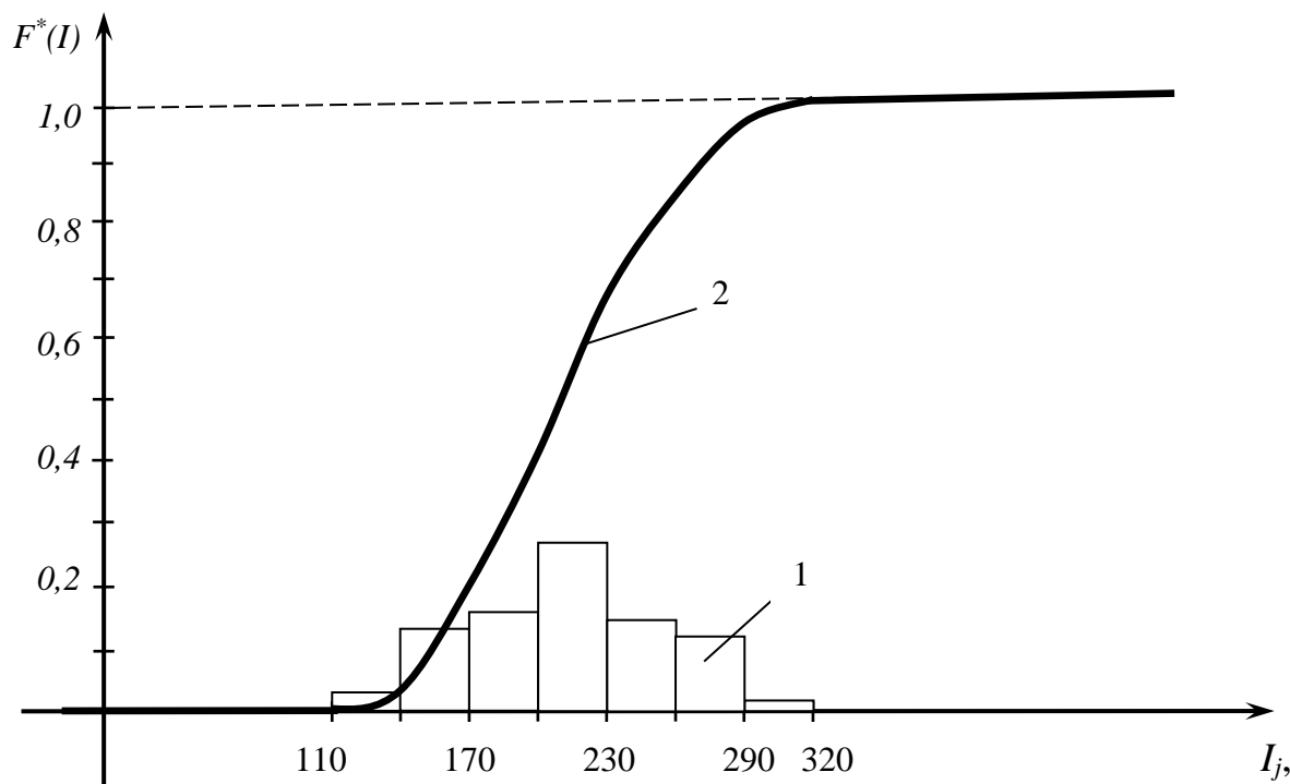
Рис. 1. Гістограма (1) і статистична функція розподілу (2) струмів витoku
