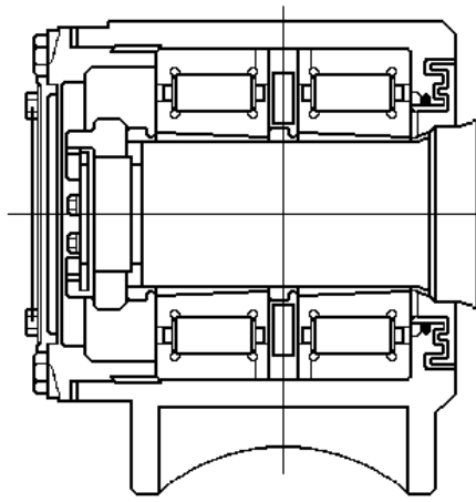
а) з двома циліндричними підшипниками
