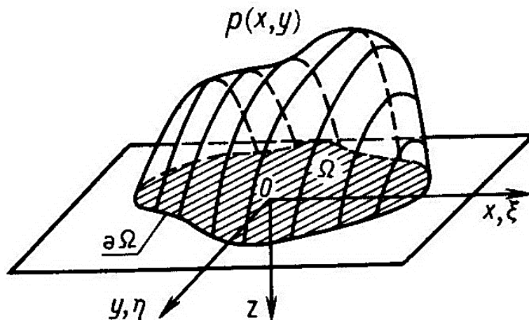
Рисунок 4.1 - Схема контакту двох поверхонь
