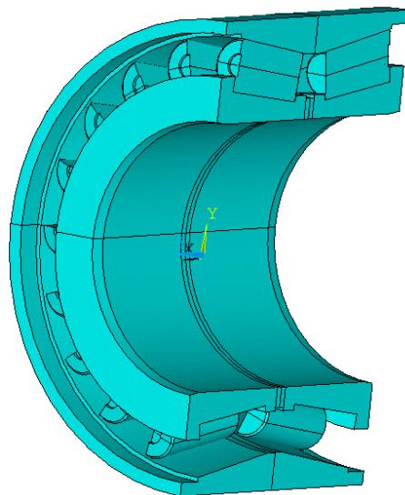
Рисунок 4.5 - Геометрична модель дворядного конічного підшипника
