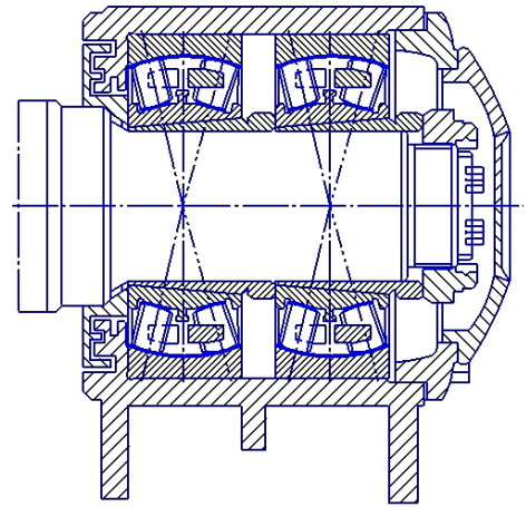
б) з двома сферичними підшипниками
