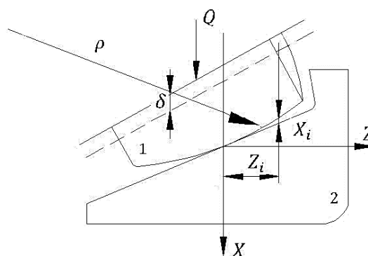
Рисунок 4.3 - Схема контакту конічного ролика з внутрішнім кільцем
