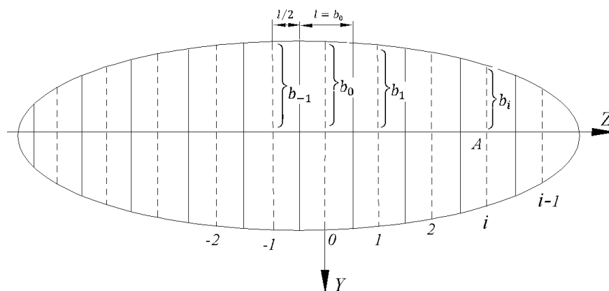
Рисунок 4.4 - Схема розбиття площадки контакту
