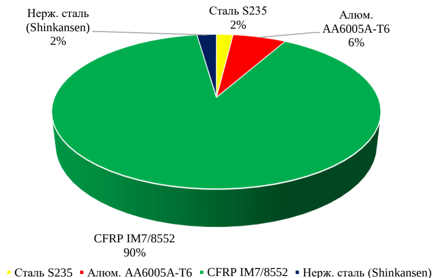
Рисунок 2.4 - Порівняння конструкційних матеріалів: питома міцність та маса носового конуса ВШС-поїзда
