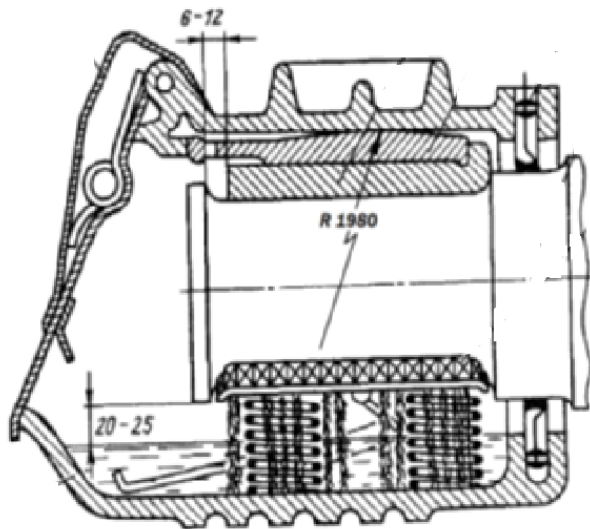
Рисунок 3.1 - Букса з підшипником ковзання
