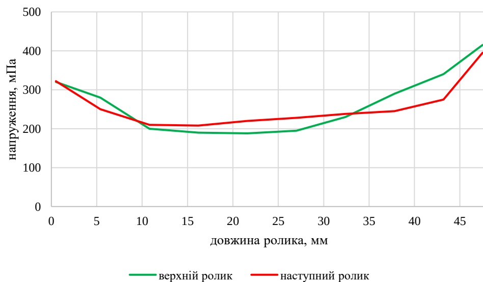
Рисунок 4.12 - Залежності зміни максимальних контактних напружень у передній зоні касетного підшипника
