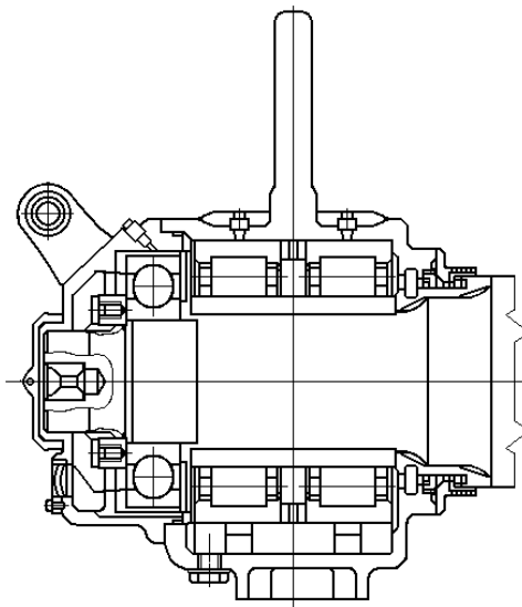
Рисунок 3.10 - Букса японського експреса Токайдо
