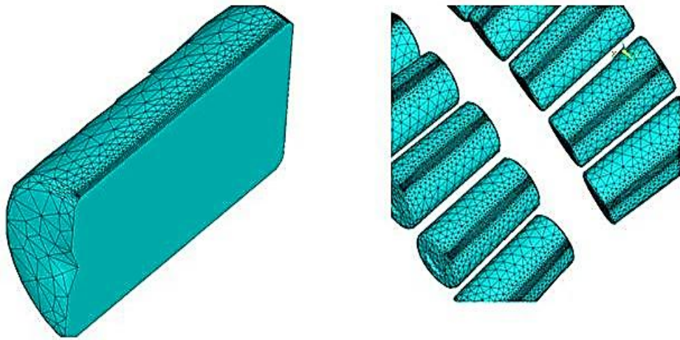
Рисунок 4.7 - Уточнення скінченно-елементної сітки в зоні контакту
