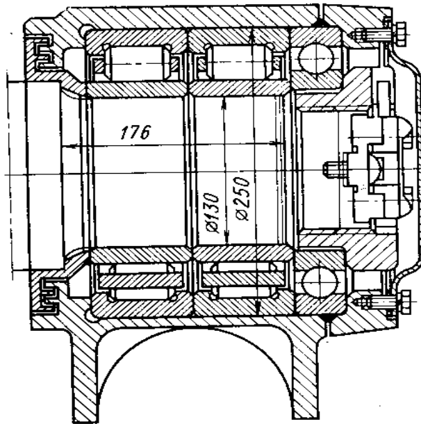
Рисунок 3.4 - Букса швидкісного поїзда Аврора
