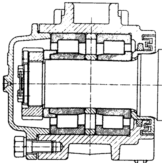
Рисунок 3.7 - Букса фірми FAG з Г-подібним упорним кільцем
