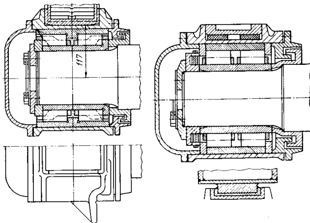
Рисунок 3.5 - Букси вагонів залізниць Польщі
