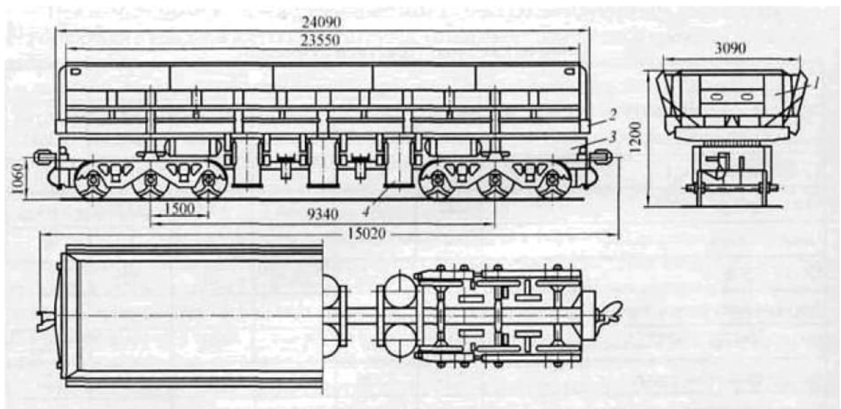
Рисунок 2.3 – Вагон-самоскид типу 2ВС-105 вантажопідйомністю 105 т
