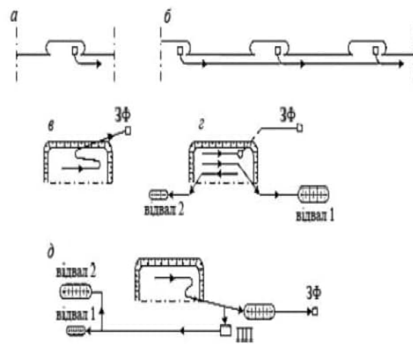
Рисунок 2.2 – Схеми кар'єрних вантажопотоків: а - елементарний, б – загальний, в – зосереджений, г – розосереджений, д – змішаний, ЗФ – збагачувальна фабрика, ПП – пункт перевантаження
