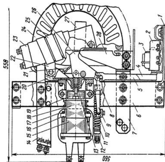
Швидкодіючий контактор БК-78Т
