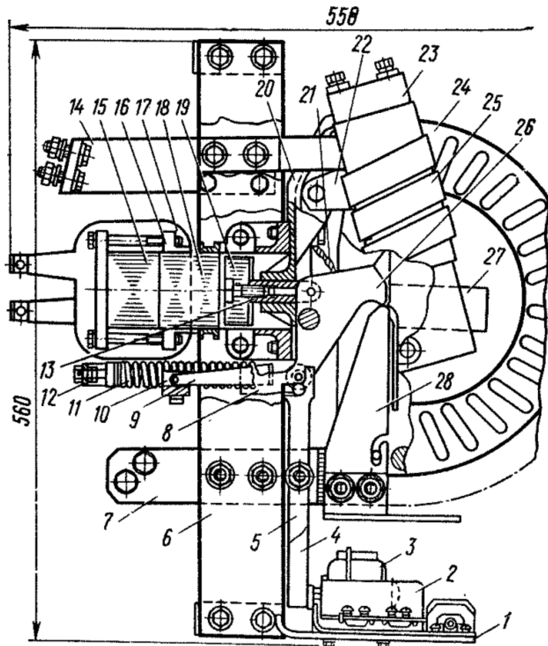
Рис. 1.8 – Швидкодіючий контактор БК-78Т
