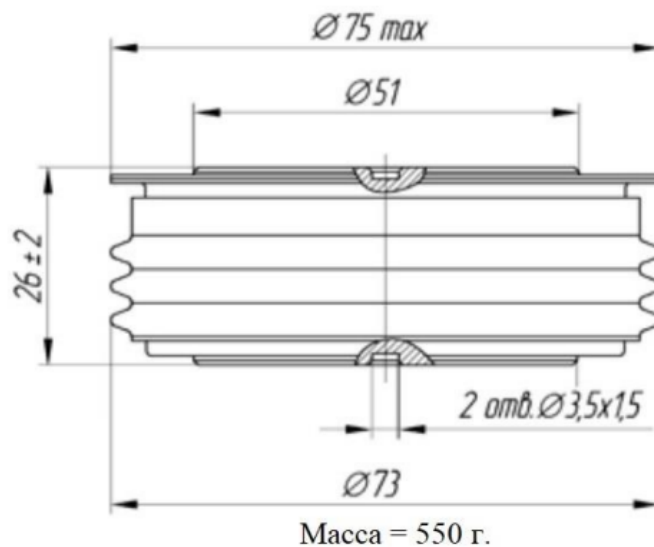
Рис. 3.11 – Масогабаритні розміри ОНС453-15
