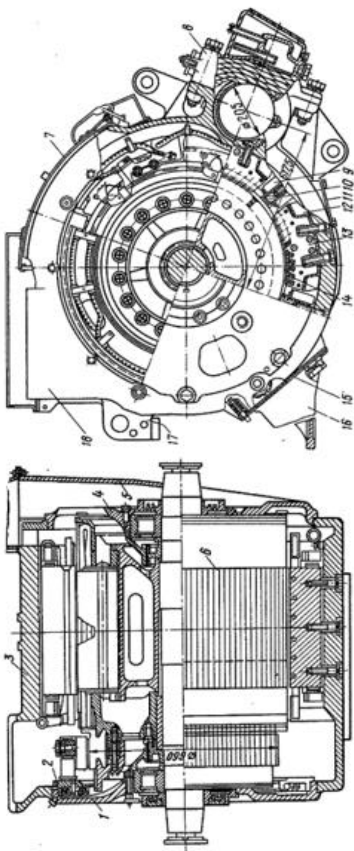
Рис. 1.6 – Тяговий електродвигун ТЛ2К1: а – поздовжній розріз; б – поперечний розріз
