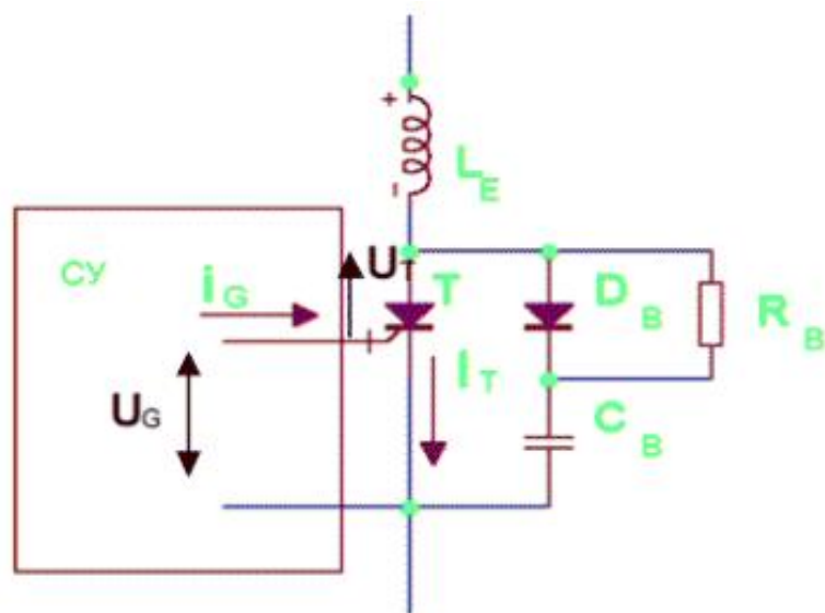
Рис. 2.3 – Схема захисного снаберного кола тиристора
