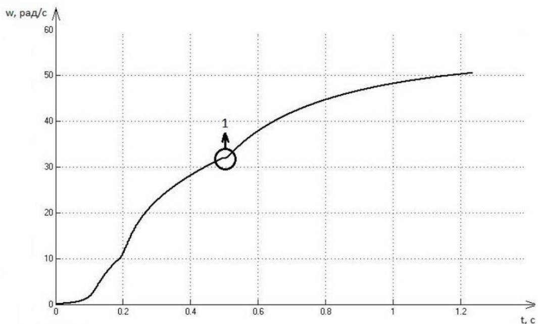
Рис. 3.4 – Графік залежності швидкості тягового електродвигуна постійного струму від часу
