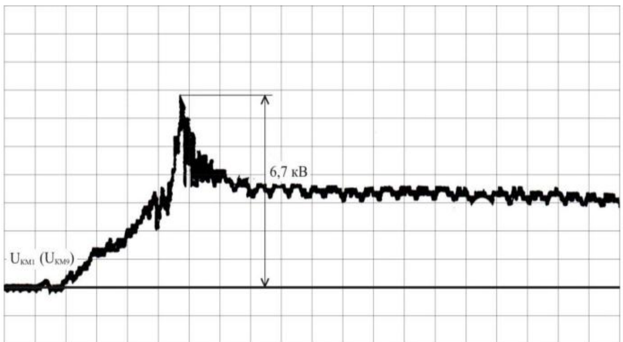
Рис. 1.10 – Осцилограма напруги при відключенні лінійного контактора КМ1 (КМ9)
