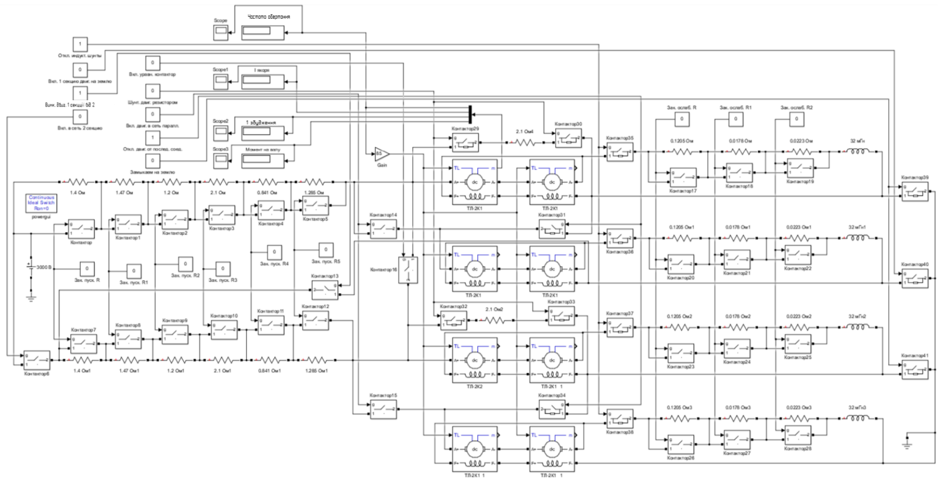
Рис. 3.2 – Електрична схема у програмному продукті Matlab Simulink
