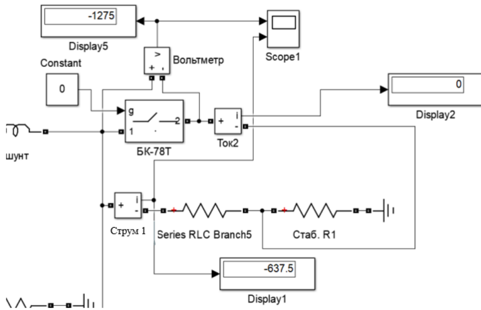
Рис. 3.17 – Схема з БК-78Т
