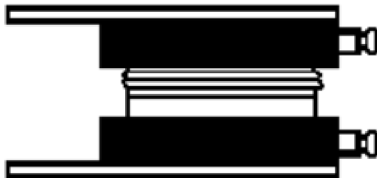
Рис. 3.9 – Профіль охолоджувача ДЖІЦ.32281.011-01
