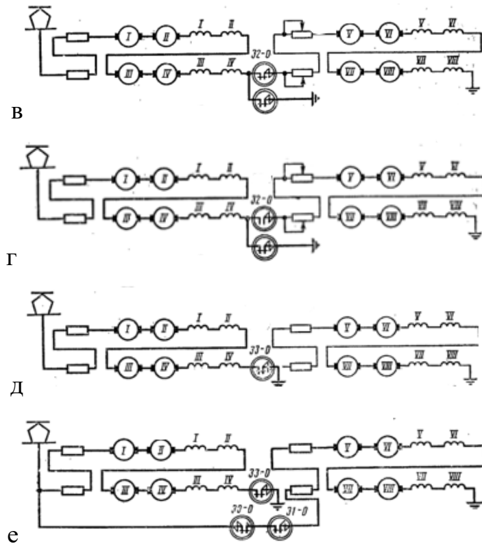
Рис. 3.3 – Схеми перемикання тягових двигунів восьмивісного електровоза з послідовного на послідовно-паралельне з'єднання: а – послідовне з'єднання; б, в, г, д, е – відповідно 1, 2, 3, 4 і 5-та перехідні позиції
