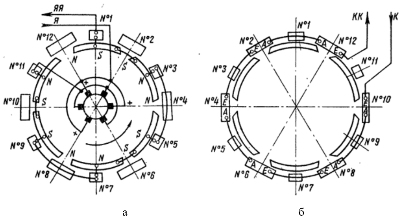
Рис. 1.7 – Схеми з'єднання котушок полюсів тягового електродвигуна ТЛ2К1: а – з боку колектора; б – з протилежного боку колектора
