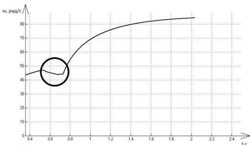
Рис. 3.9 – Графік залежності швидкості тягового електродвигуна постійного струму від часу
