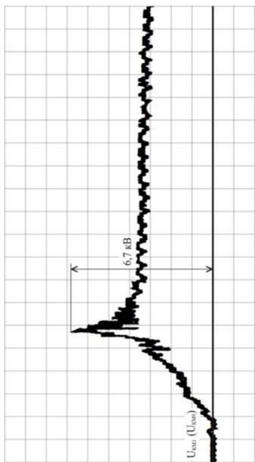
Осцилограма напруги при відключенні лінійного контактора КМ1 (КМ9)
