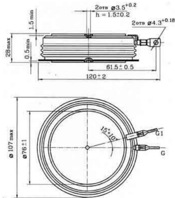
Рис. 3.8 – Запираючий силовий тиристор ТЗЗ73-2000
