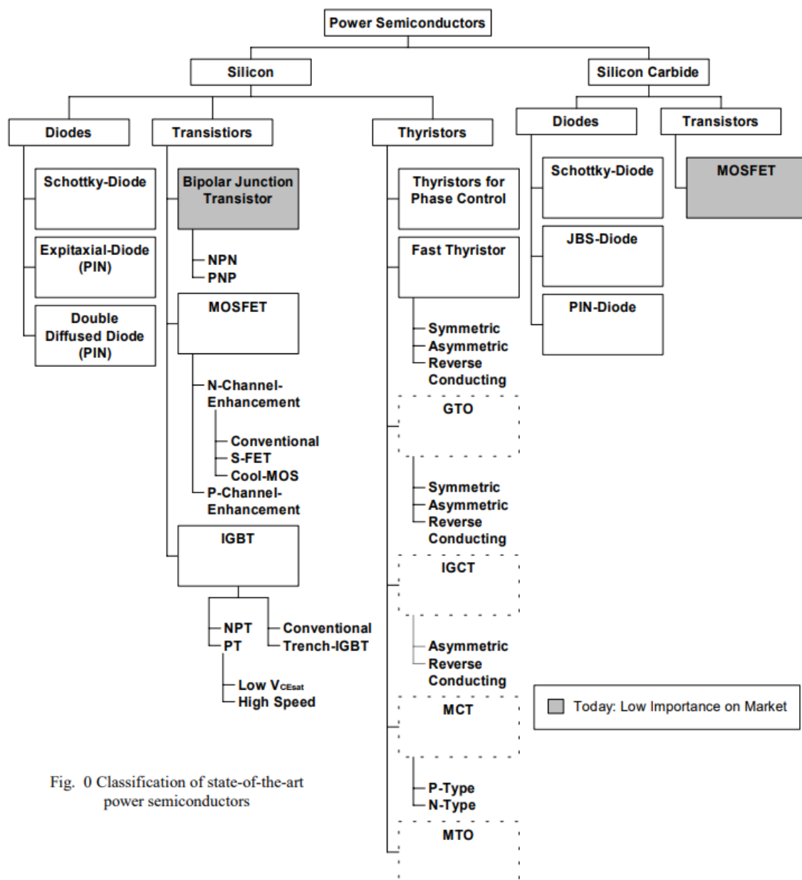
Рис.2.1 – Класифікація силових напівпровідникових ключів
