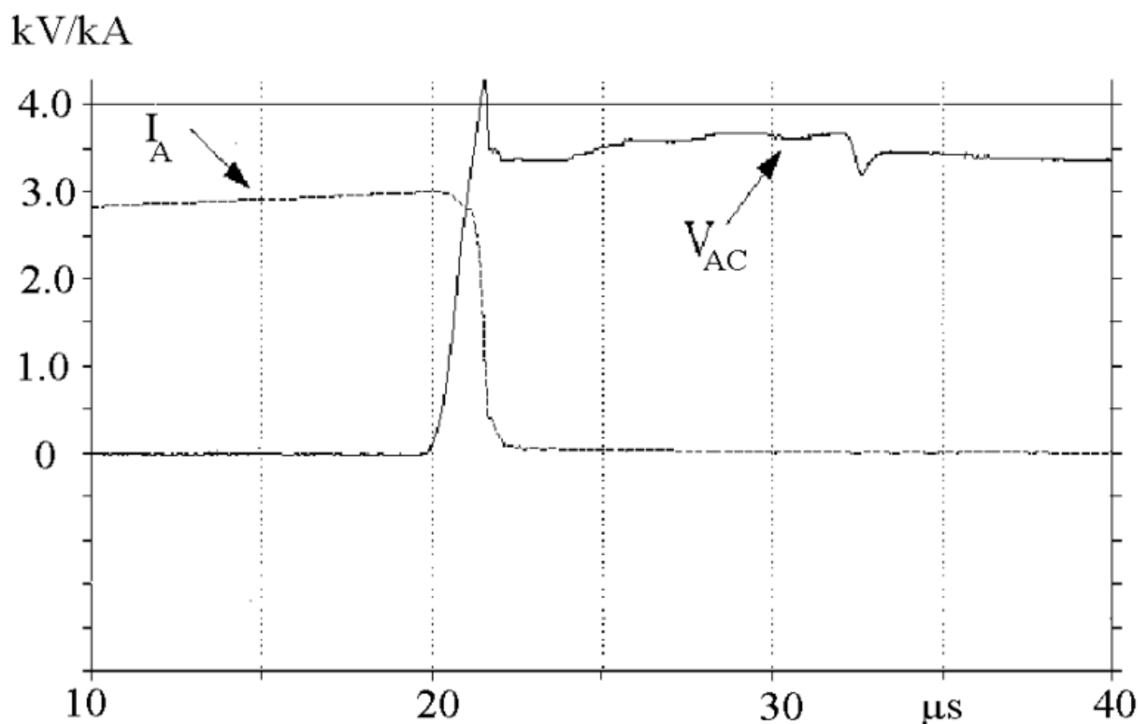
Рис.2.3 – Осцилограмма комутації запираємого тиристора типу 5SGX 06F6004 ( V_{dc-link} = 3.3\text{kV} , T_j(t = 0) = 80^\circ\text{C} , L_r = 17\mu\text{H} , \text{Load} = 2\text{mH}/50\text{ m}\Omega , t_{on} = 10\text{ }\mu\text{s} , t_{off} = 30\text{ }\mu\text{s} )
