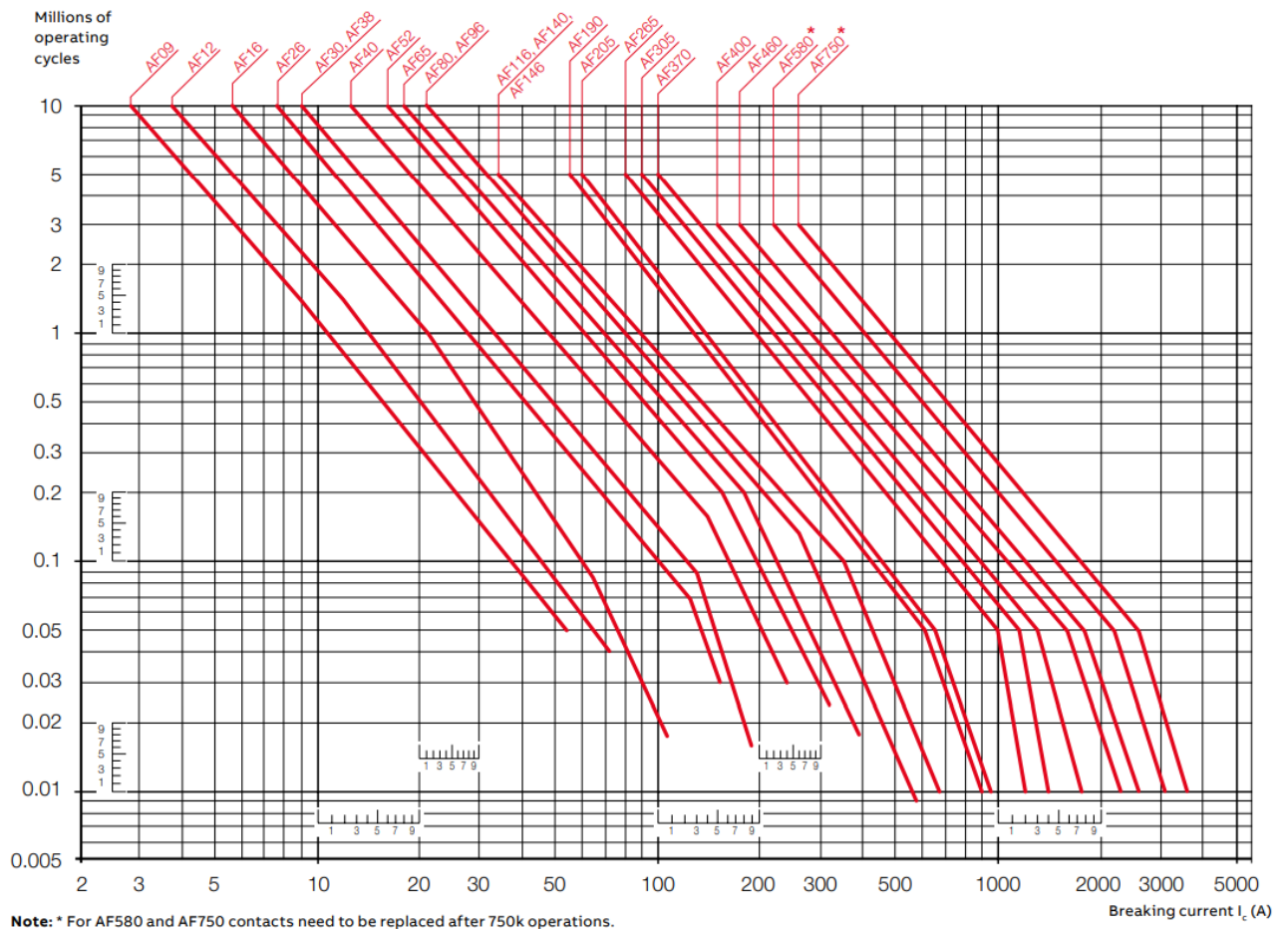
Рис.1.11 – Показники надійності силових контакторів АВВ:
