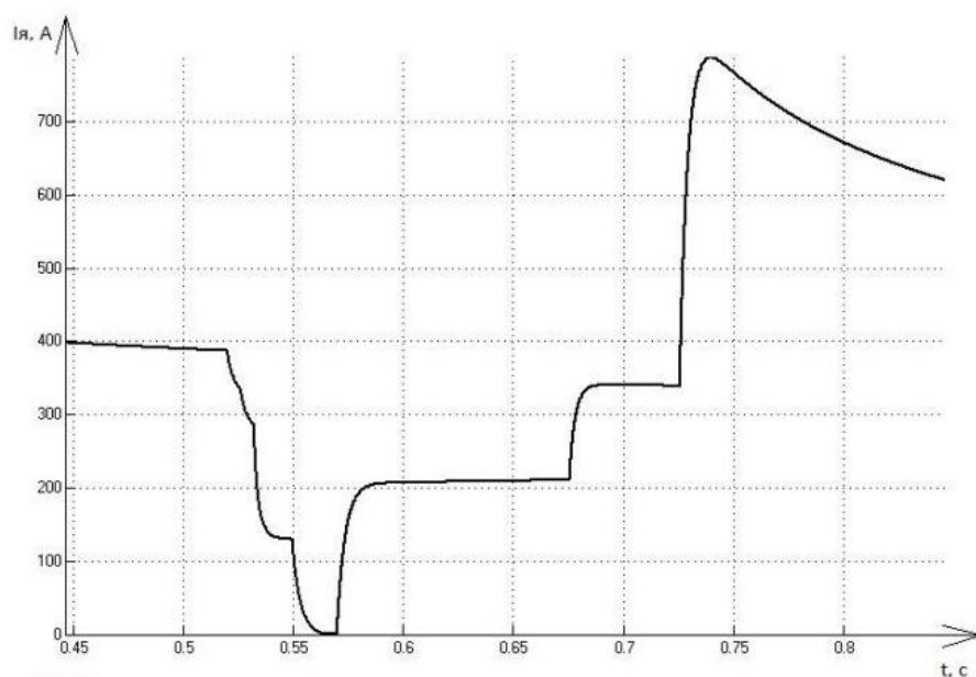
Рис. 3.10 – Графік залежності струму якоря від часу
