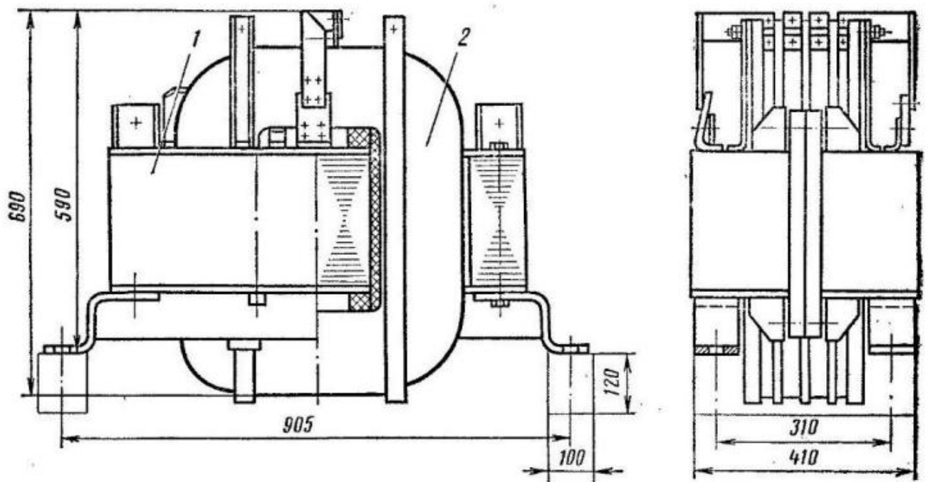
Рис. 3.14 – Індуктивний шунт ИШ-2К
