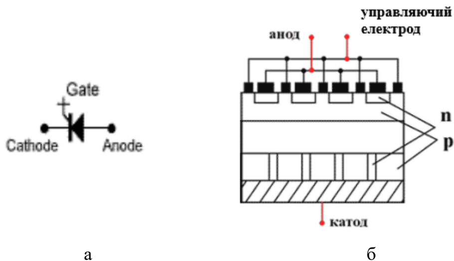
Рис. 2.1 – Замикаючий тиристор: а – умовне позначення; б - структурна схема
