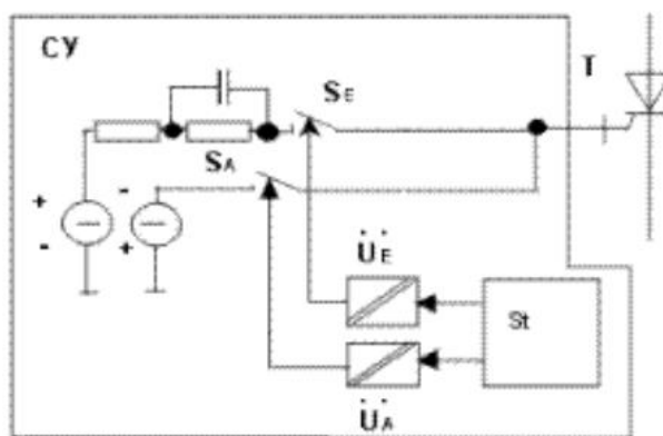
Рис. 2.4 – Один із варіантів ланцюга управління
