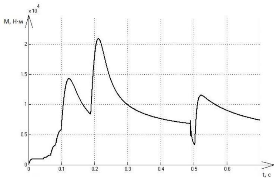
Рис. 3.7 – Графік залежності моменту на валу від часу моделювання
