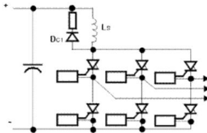
Рис. 2.6 – Схема трифазного інвертора на IGCT тиристорах
