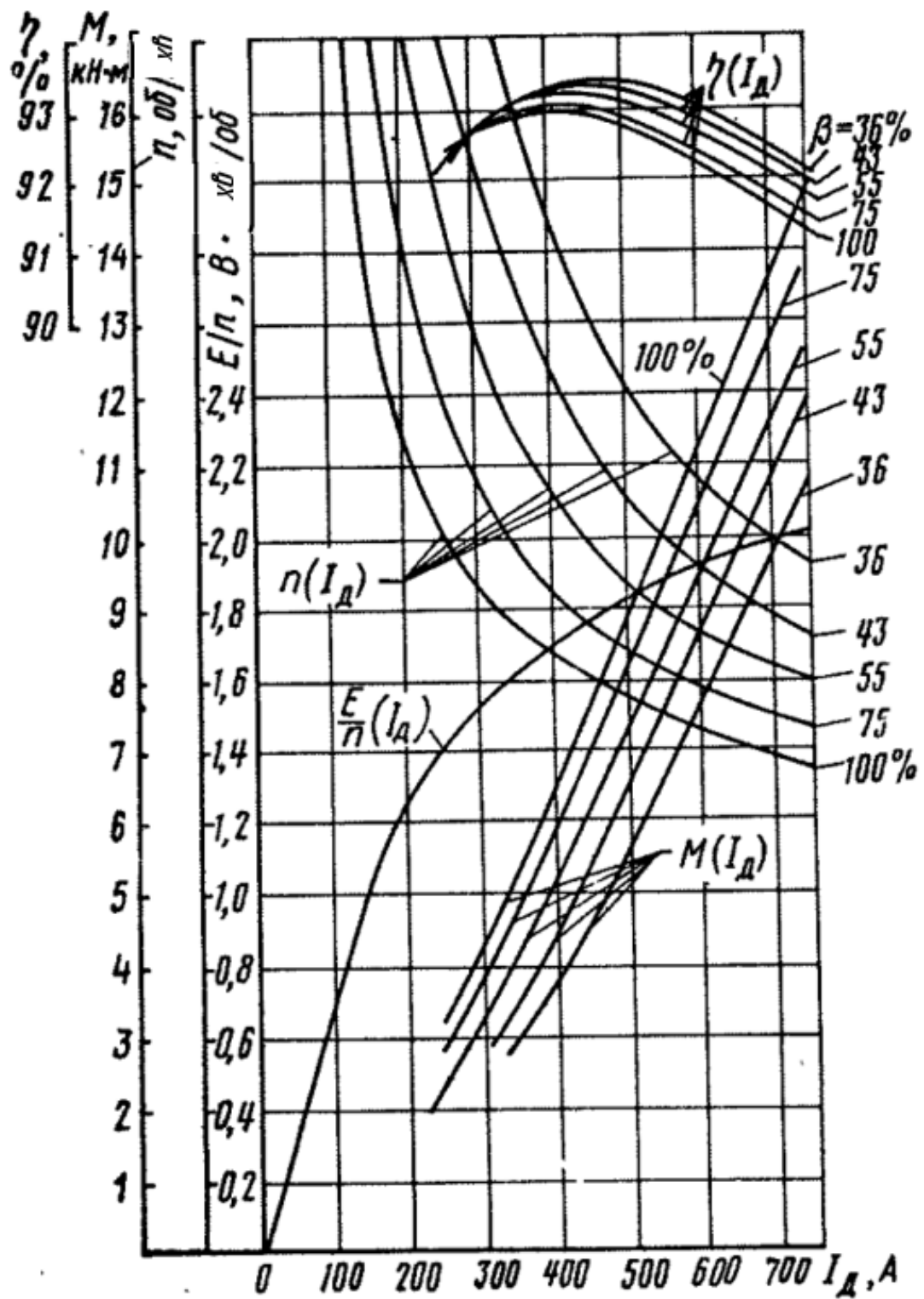
Рис. 1.5 – Електромеханічні характеристики тягового електродвигуна ТЛ2К1 при U_d = 1500 В
