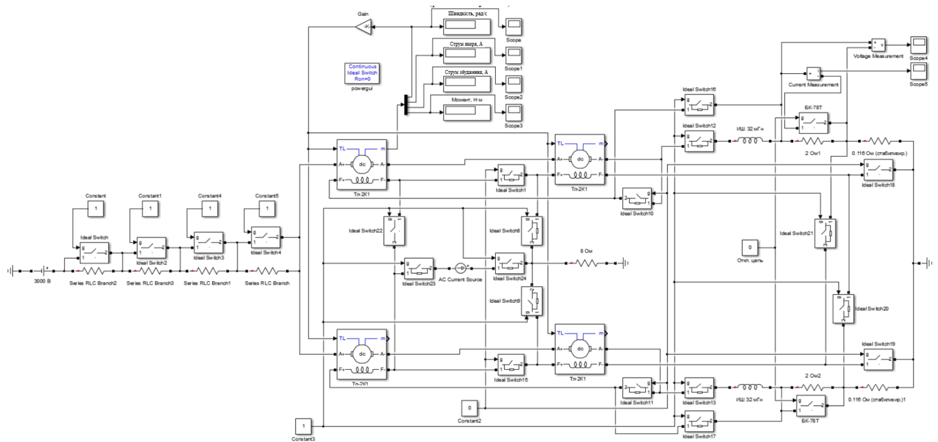
Рис. 3.16 – Електрична схема РКСУ електровоза в режимі рекуперації у програмному продукті Matlab Simulink
