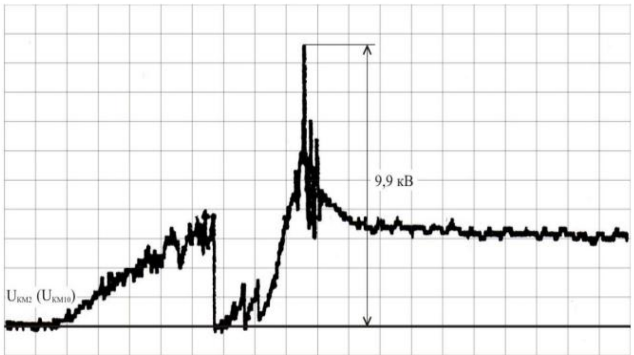
Рис. 1.9 – Осцилограма напруги при відключенні контактора КМ2 (КМ10)
