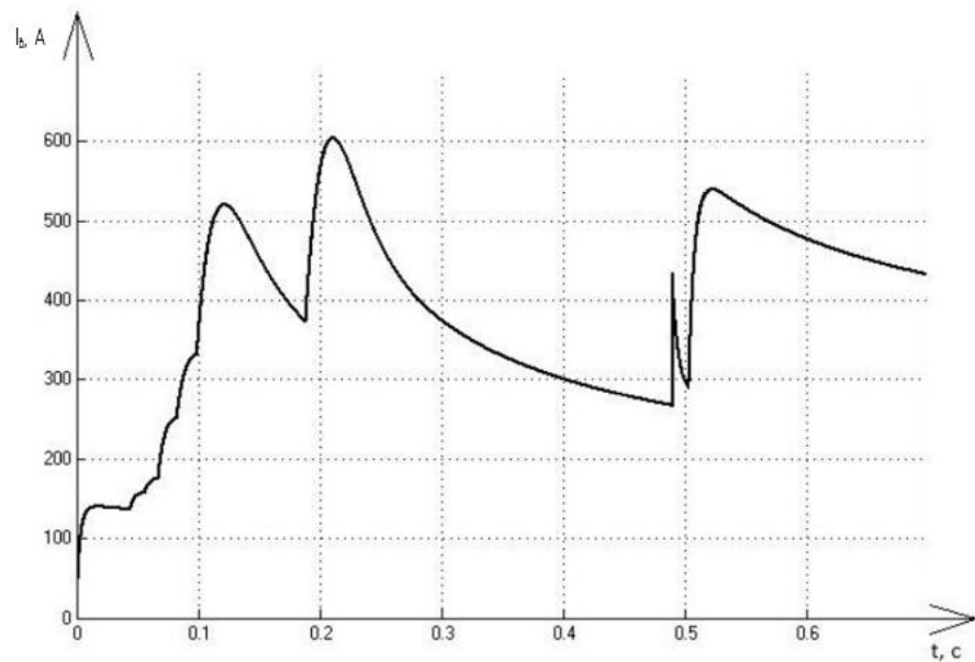
Рис. 3.6 – Графік залежності струму збудження від часу моделювання
