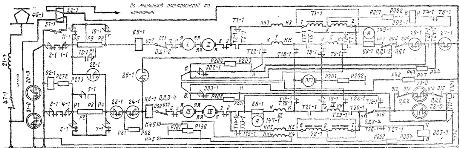
Рис. 3.15 – Схема силового ланцюга при рекуперативному режимі гальмування на паралельному з'єднанні обмоток якорів тягових двигунів під час руху вперед електровозів ВЛ10 та ВЛ10 у
