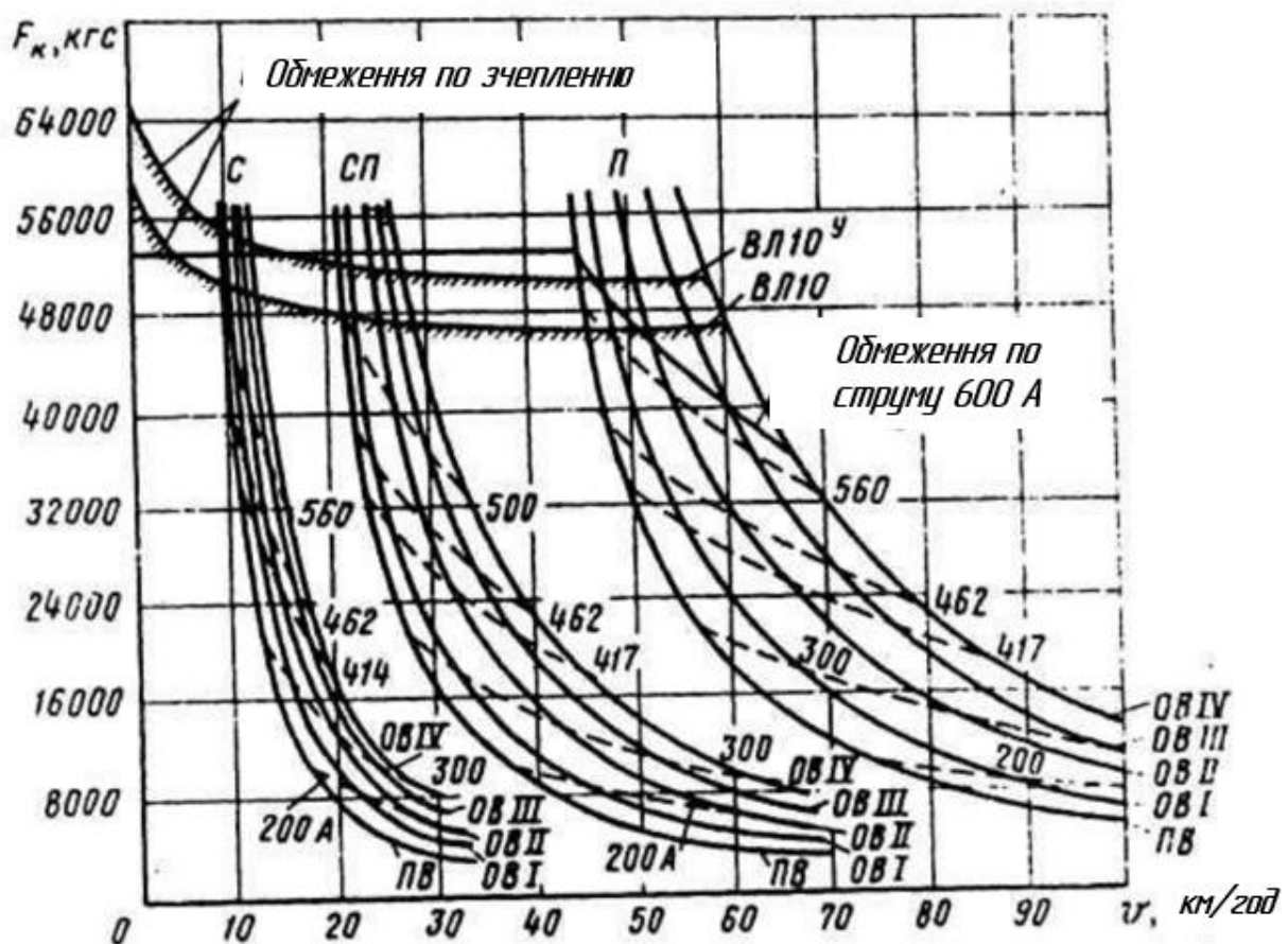
Рис. 1.3 – Тягові характеристики електровозів серії ВЛ10 та ВЛ10 у
