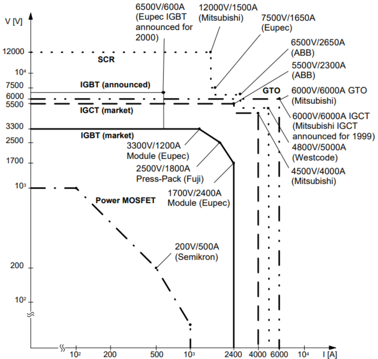
Рис.2.2 – Діапазон можливих значень комутованих струмів та напруг сучасних напівпровідникових ключів
