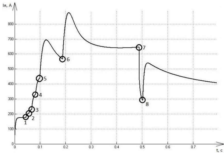
Рис. 3.5 – Графік залежності струму якоря від часу
