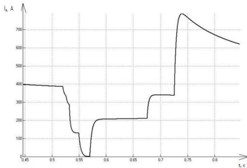
Рис. 3.11 – Графік залежності струму збудження від часу
