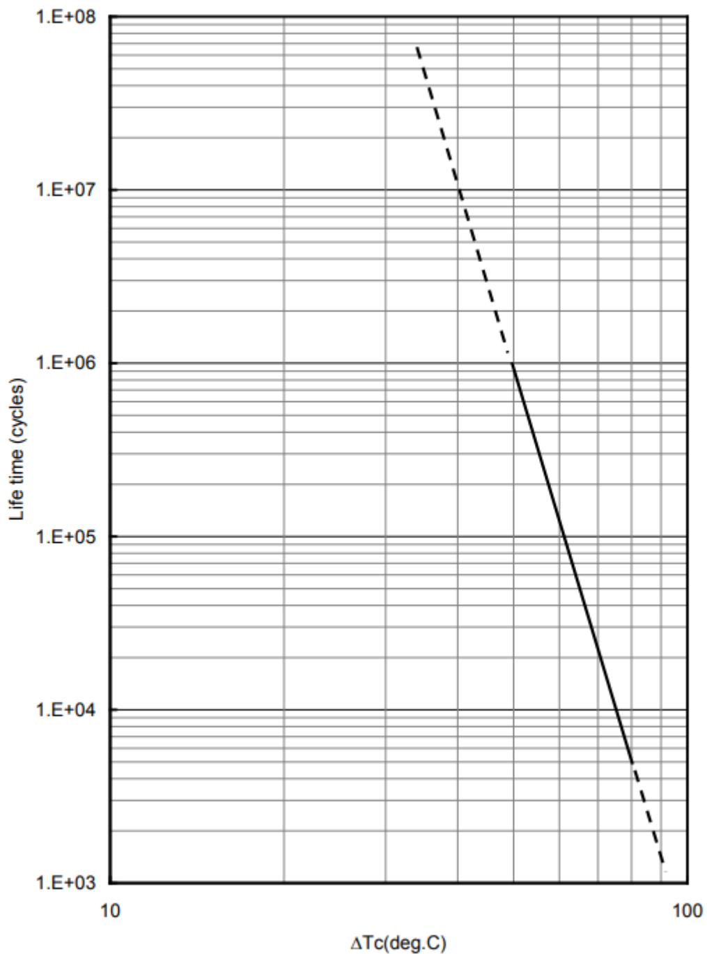
Рис.2.7 – Залежність числа комутацій IGCT комутатора від температури
