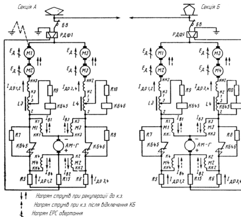
Рис. 3.13 – Схема захисту тягових електродвигунів від струмів короткого замикання в рекуперативному режимі на паралельному з'єднанні
