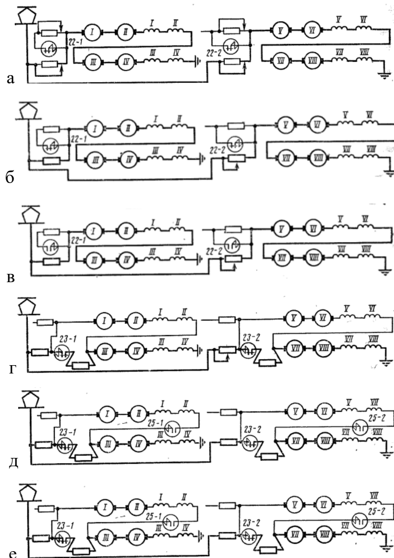
Рис. 3.8 – Схема перемикання тягових восьмиівісних двигунів електровоза з послідовно-паралельного на паралельне з'єднання: а – послідовне з'єднання; б, в, г, д, е – відповідно 1, 2, 3, 4 і 5-та перехідні позиції
