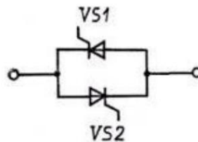
Рис. 3.7 – Схема включення тиристорів
