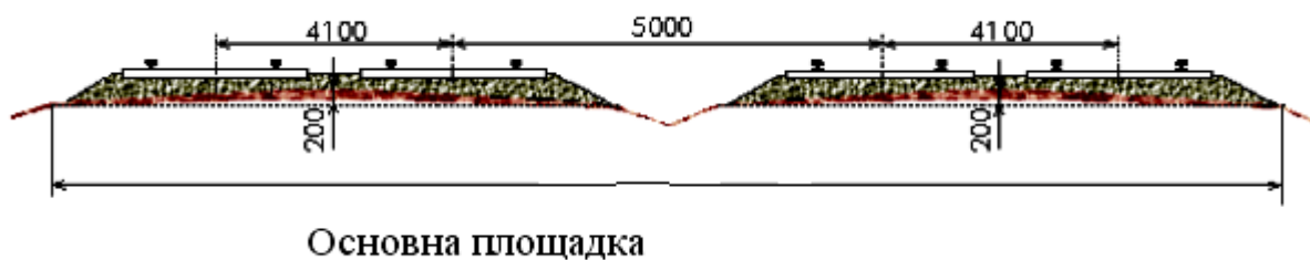
Рисунок 3 – Відстань між осями колій на перегонах
