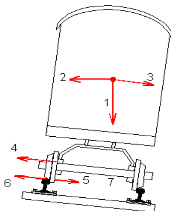
Рисунок 10 – Схема сил, що діють у кривій
