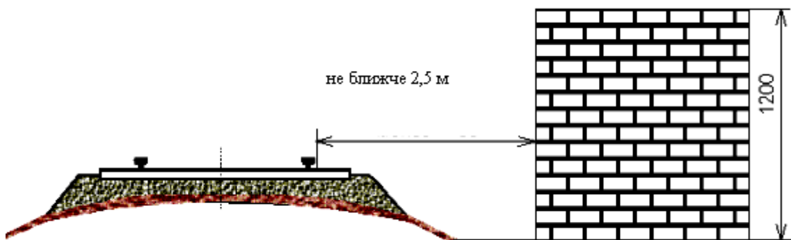
Рисунок 5 – Відстань від крайньої рейки при висоті вантажу до 1200 мм
