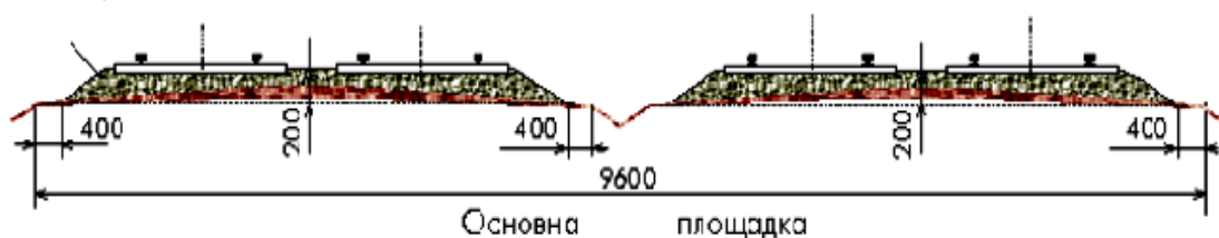
Рисунок 9 – Розміри земляного полотна двоколійної лінії
