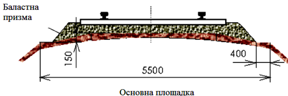
Рисунок 8 – Розміри земляного полотна одноколійної лінії
