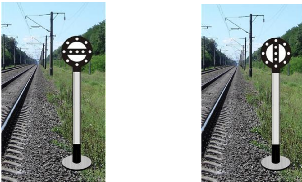
Рисунок 13 – Постійні сигнальні знаки початку та кінця небезпечного місця
