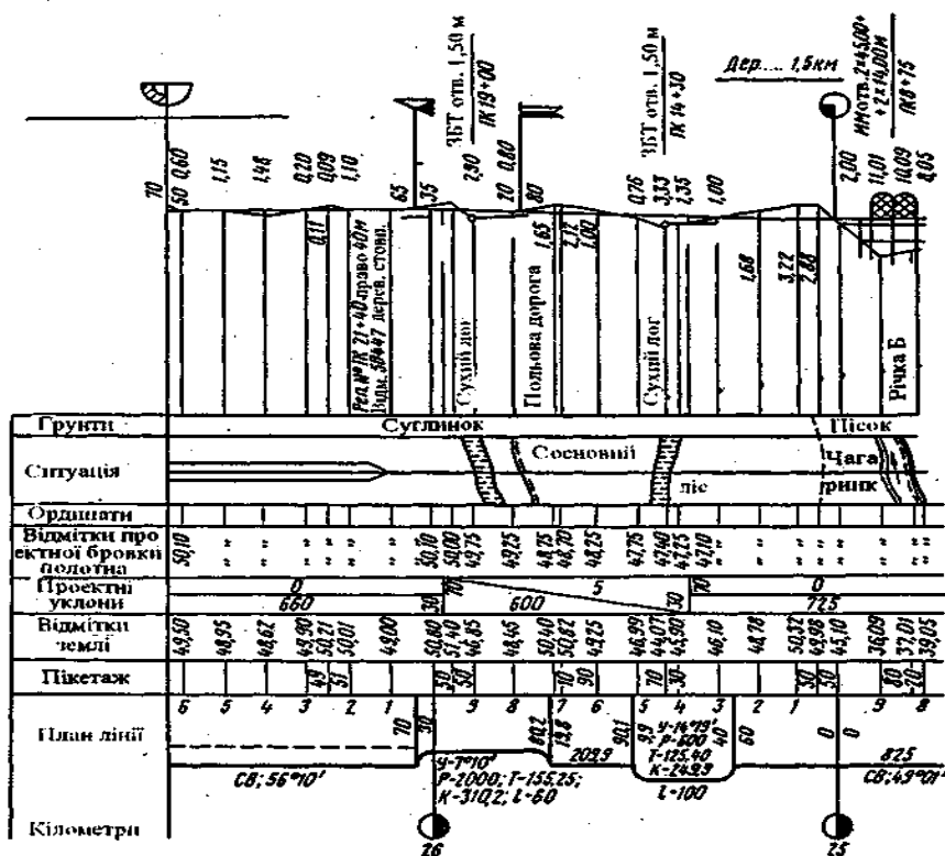
Рисунок 7 – Нормальний профіль колії
