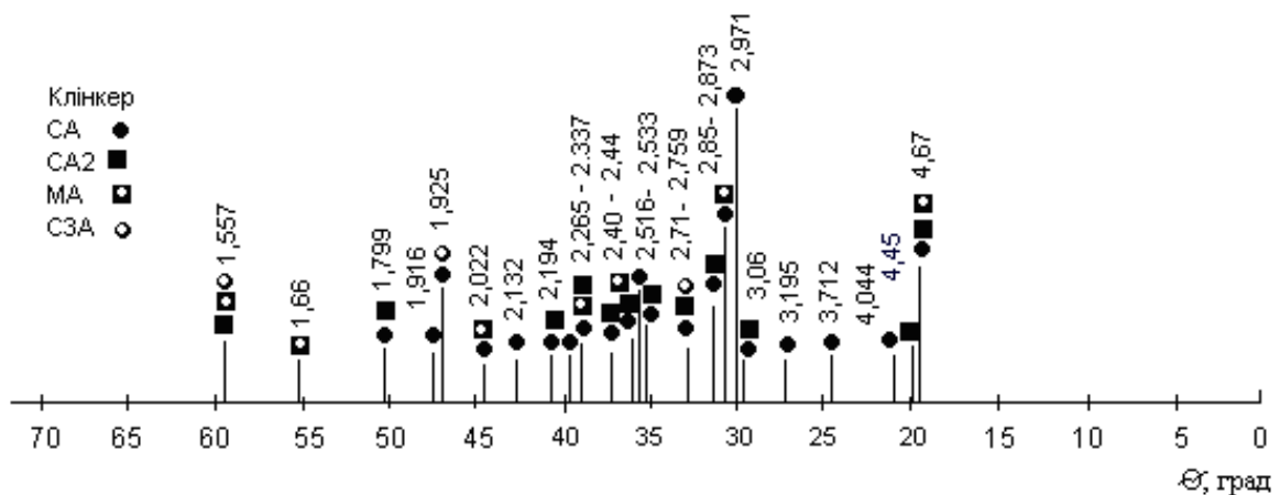
Рис. 2. Рентгенограма клінкеру
